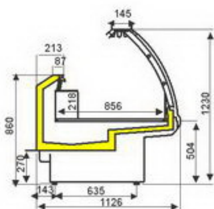
JASMINE RCA 125 (ET -10°C, 740W)
