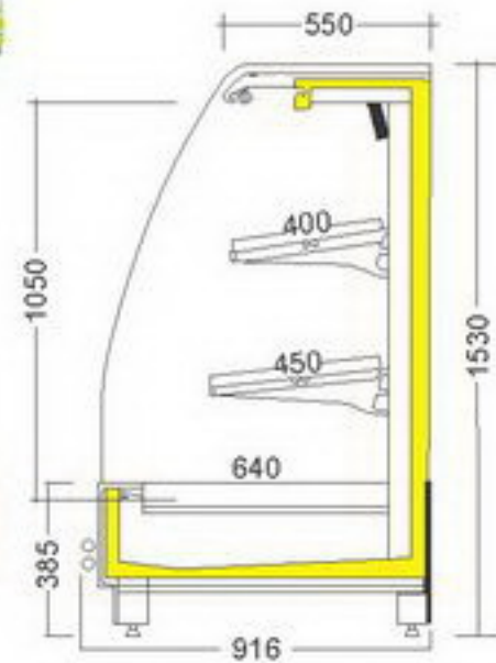
MINI MAGNOLIA ED 250CM (ET -10°C, 2900W)
